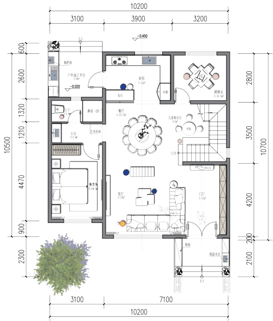
一层平面图 ▲
