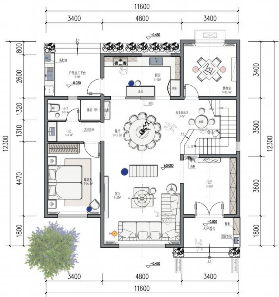
一层平面图 ▲
