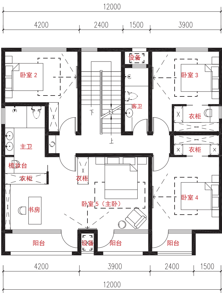
二层平面图 ▲
