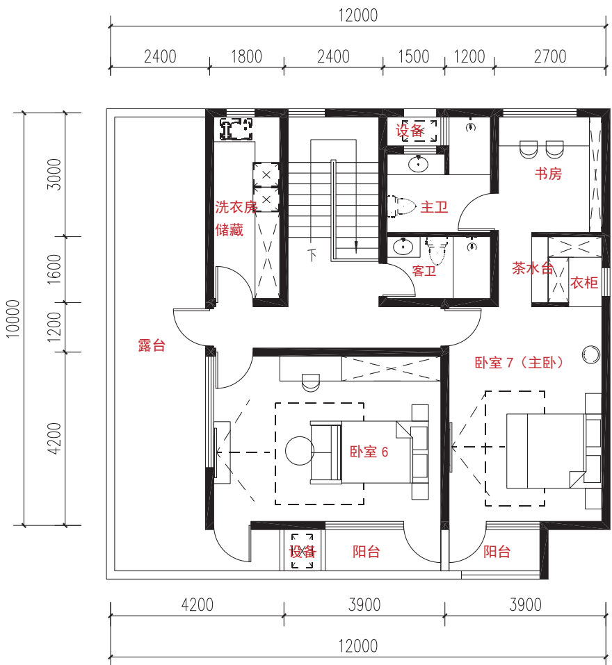
三层平面图 ▲
