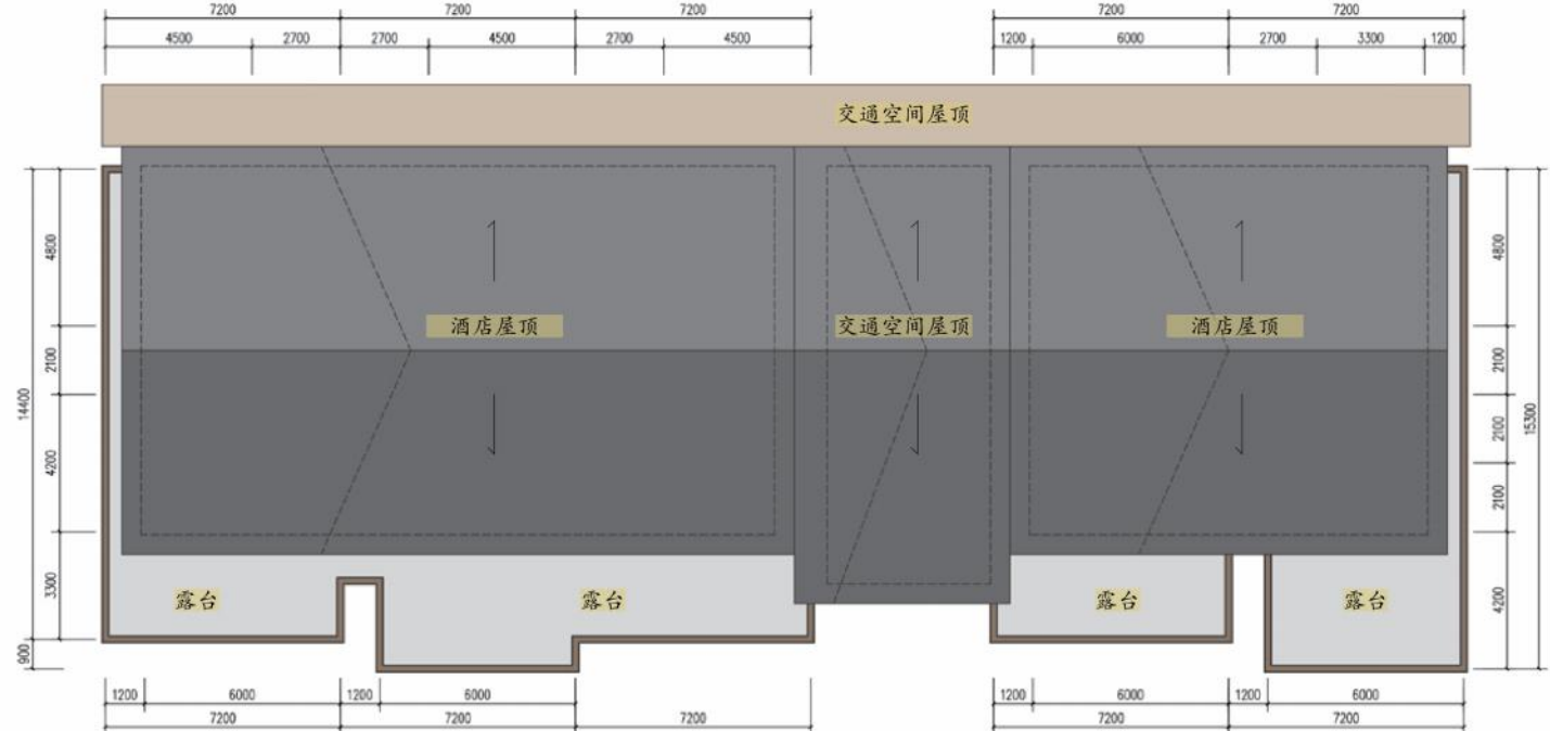
整体屋顶平面图
